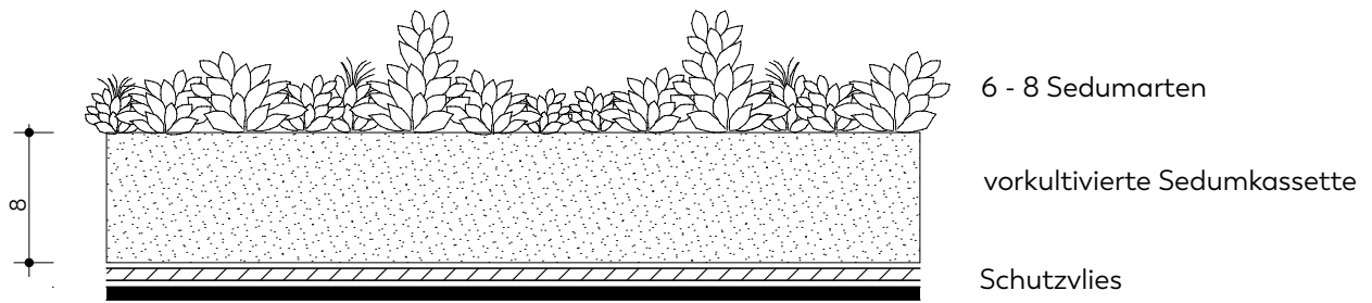
Dachaufbau mit EPDM-Abdichtung
